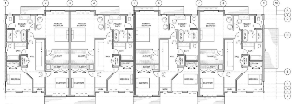
3 LEVEL 2 PLAN Scale: 1/8" = 1'-0"
