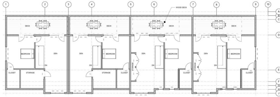
1 LEVEL 3 PLAN Scale: 1/8" = 1'-0"
